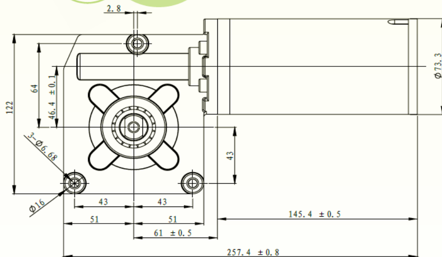
电机参数表 / Data Sheet Of 73WJS
