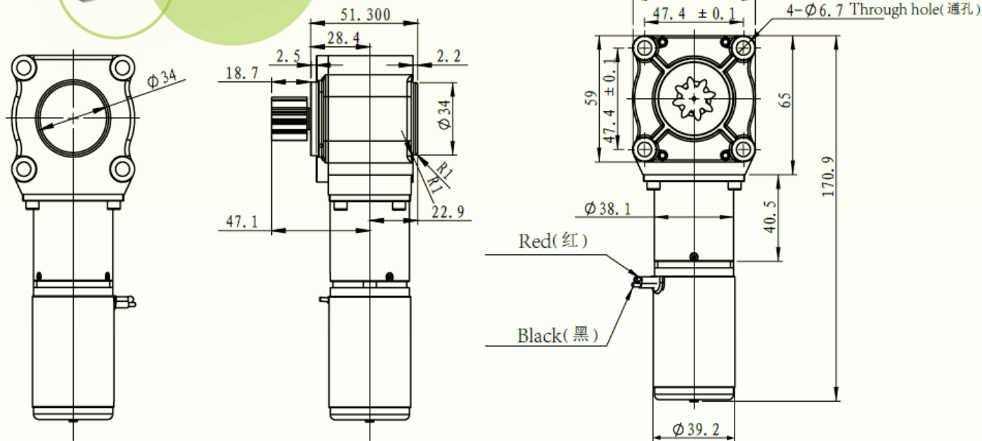
电机参数表 / Data Sheet Of 39ZYJ
