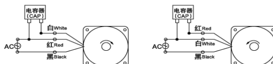
YN 型可逆电动机: REVERSIBLE MOTOR
