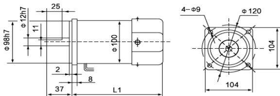
齿轮减速电机: GEAR MOTOR
