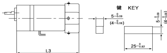
齿轮减速电机: GEAR MOTOR
