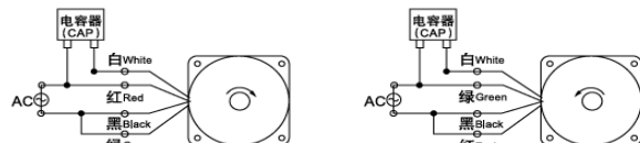
YY 型感应电动机: INDUCTION MOTOR
