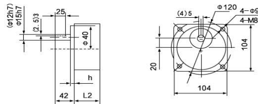
齿轮减速电机: GEAR MOTOR
