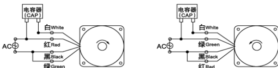
YY 型感应电动机: INDUCTION MOTOR
