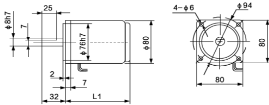
齿轮减速电机: GEAR MOTOR
