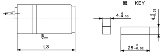
齿轮减速电机: GEAR MOTOR
