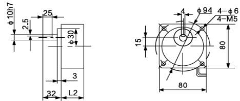
齿轮减速电机: GEAR MOTOR
