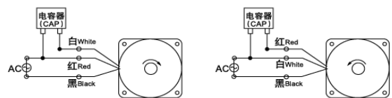
YN 型可逆电动机: REVERSIBLE MOTOR
