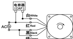
YY 型感应电动机: INDUCTION MOTOR
