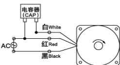
YN 型可逆电动机: REVERSIBLE MOTOR
